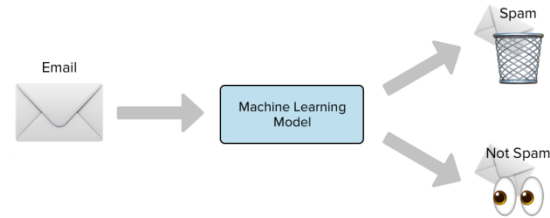
Fig.1. Data image.
