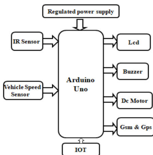
Fig1 : Block Diagram
